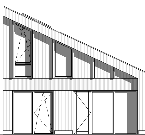
Achtergevel
