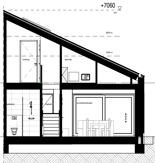
Doorsnede A
