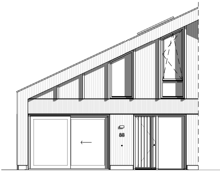
Voorgevel
